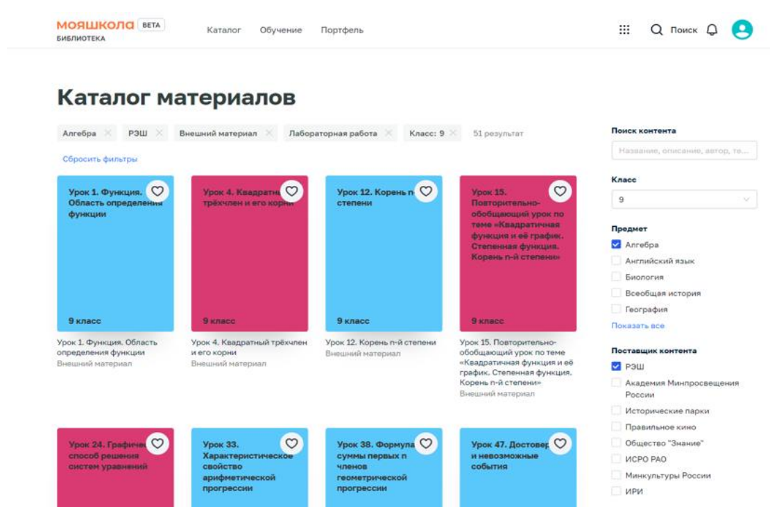
Рисунок 14. Сервис «Библиотека»
